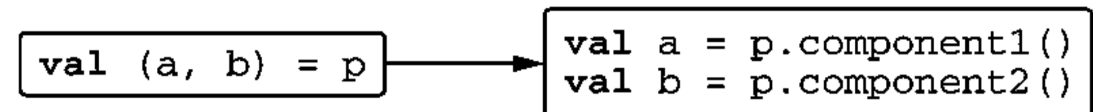
Рис. 7.10. Мультидекларация транслируется в вызовы функций componentN
