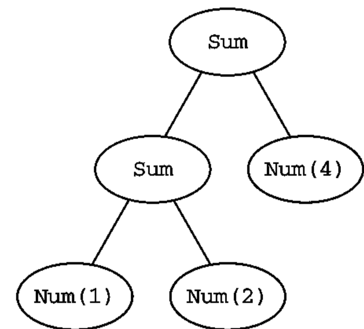
Рис. 2.4. Представление выражения Sum(Sum(Num(1), Num(2)), Num(4))
