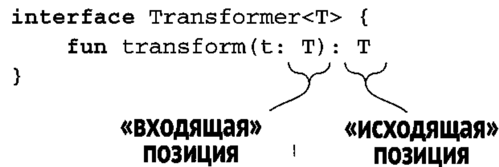
Рис. 9.6. Тип параметра функции называют входящей позицией, а тип возвращаемого значения – исходящей
