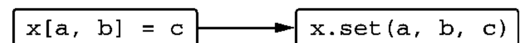
Рис. 7.7. Операция присваивания с применением квадратных скобок транслируется в вызов функции set
