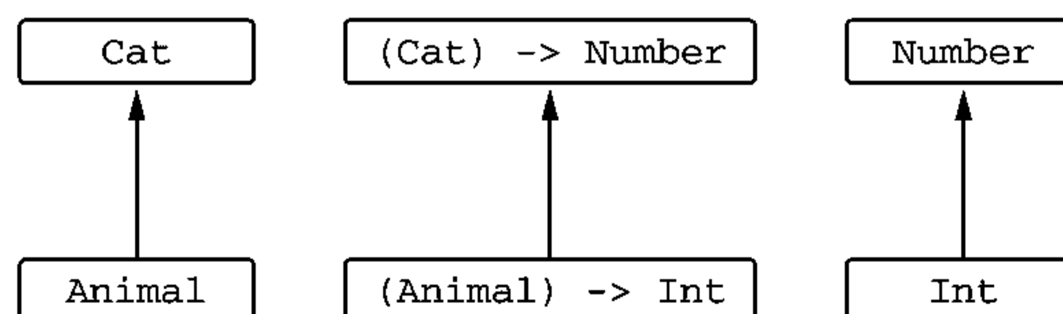
Рис. 9.8. Функция (T) \rightarrow R контравариантна по своему аргументу и ковариантна по типу возвращаемого значения
