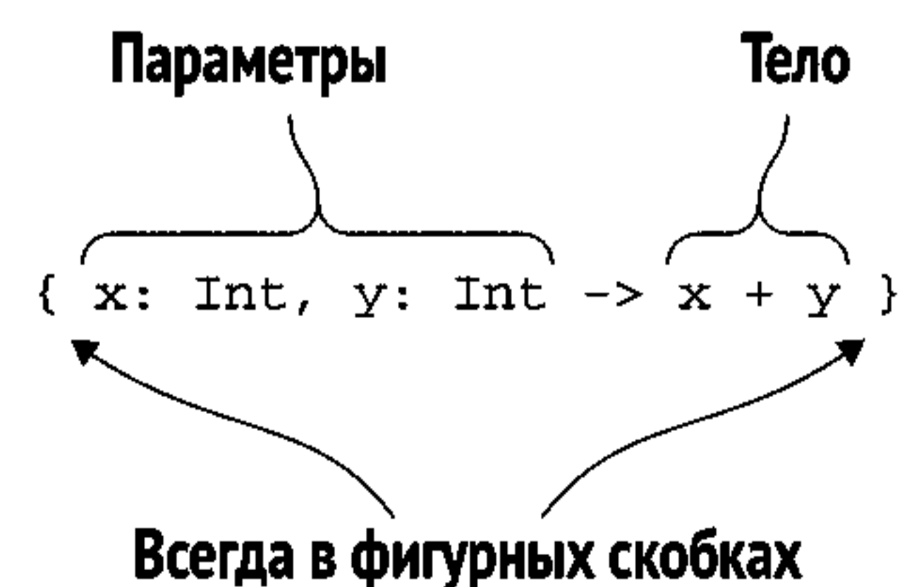
Рис. 5.1. Синтаксис лямбда-выражений
