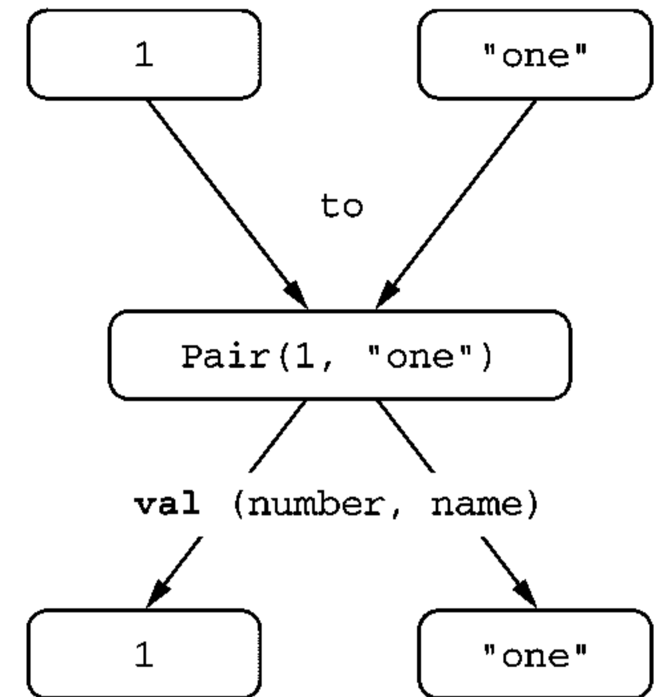
Рис. 3.3. Создание пары с помощью функции to и её распаковка с помощью мультидекларации
