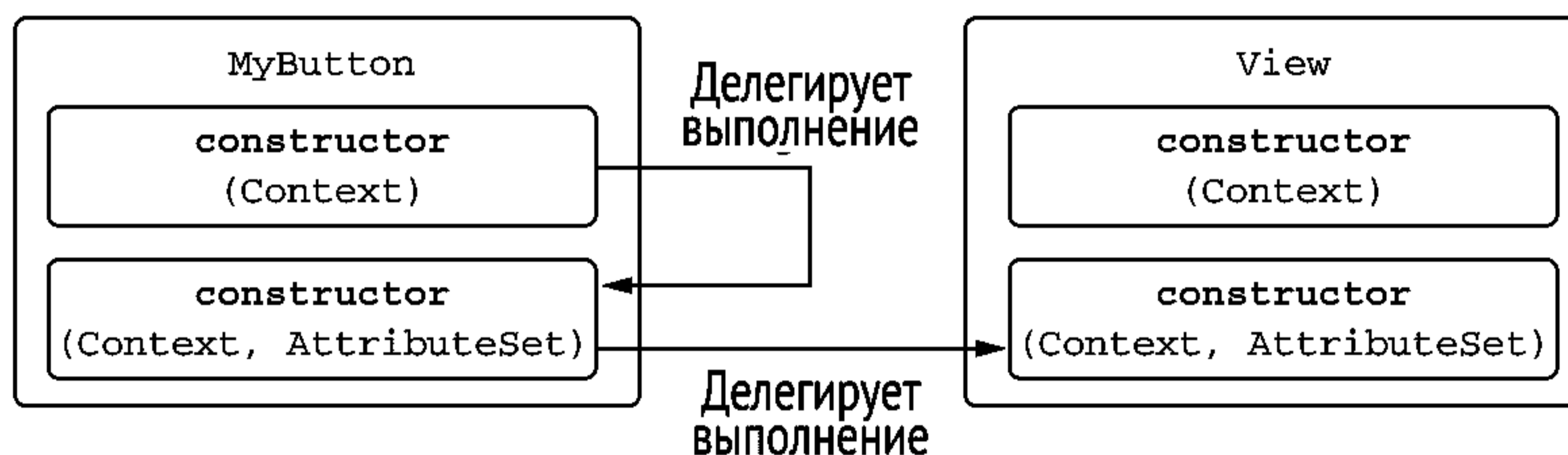
Рис. 4.4. Делегирование выполнения конструктору того же класса
