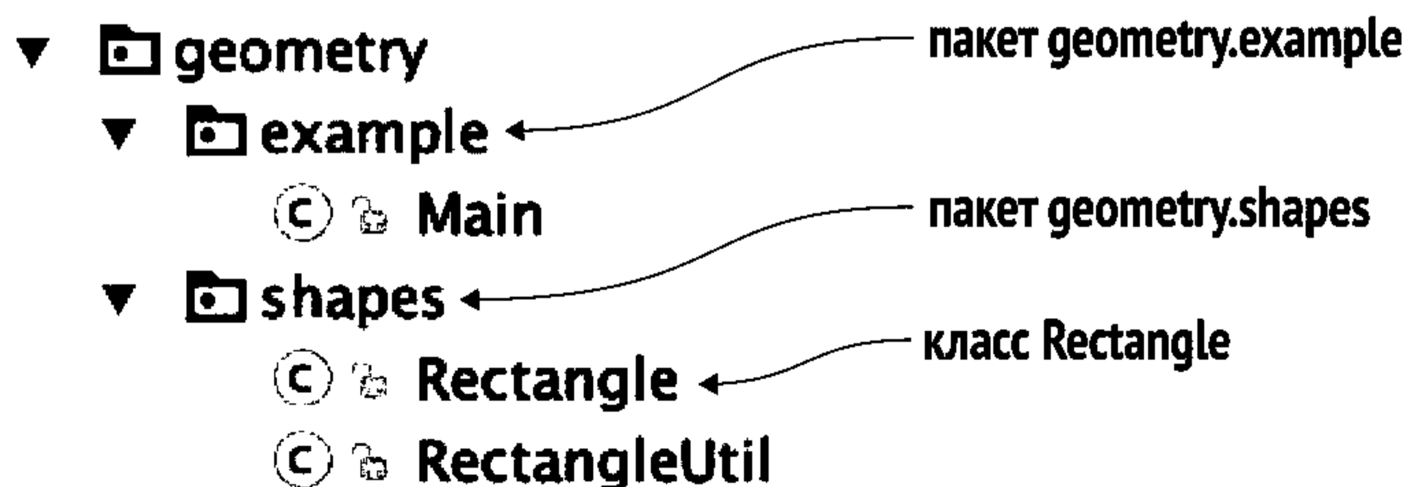
Рис. 2.2. В Java иерархия каталогов соответствует иерархии пакетов
