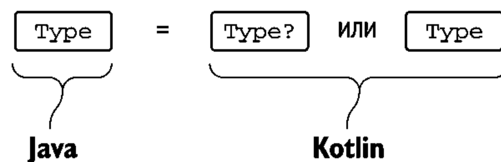
Рис. 6.9. Типы Java представлены в Kotlin как платформенные типы, которые могут поддерживать или не поддерживать значение null
