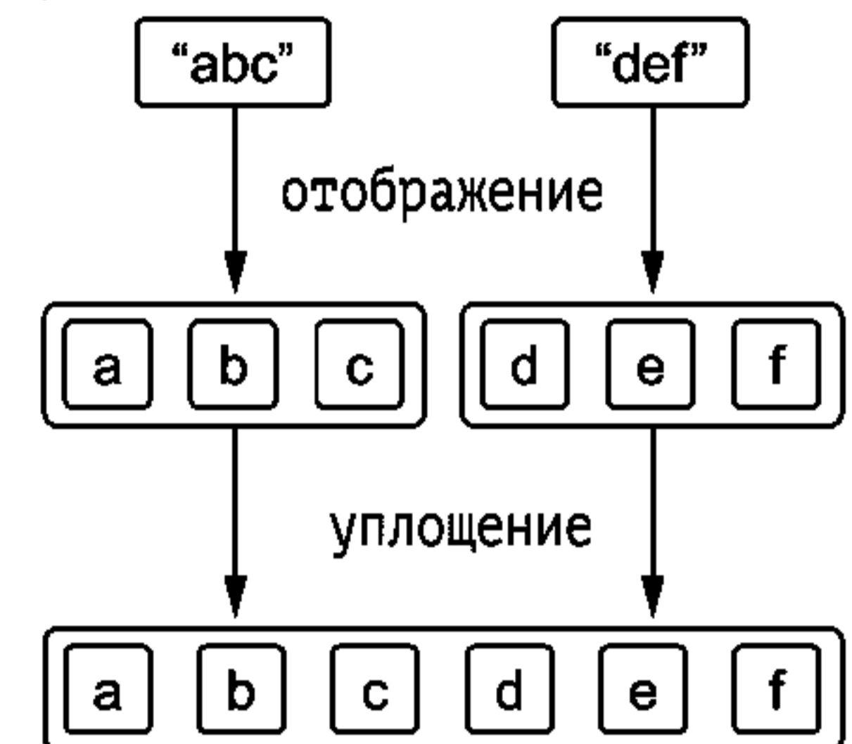
Рис. 5.6. Результат применения функции flatMap
